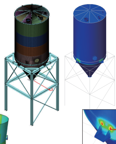
応力集中
