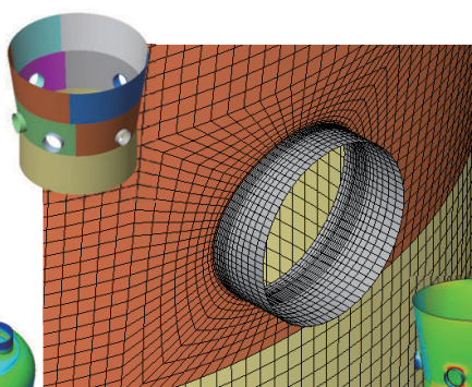
Quadrilateral Mesh
