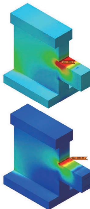
引張主応力
