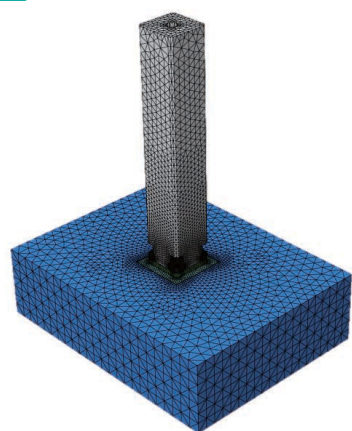
全体モデル
