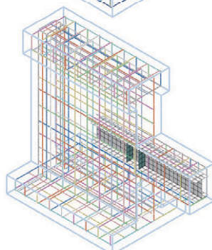
解析モデル
